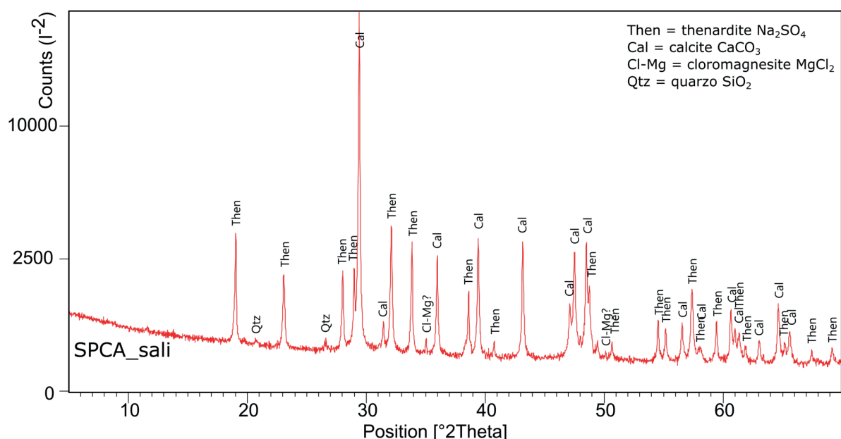
Fig. 9 - Diffattogramma dell'analisi XRD del campione di efflorescenze (SPCA) prelevate dalla superficie del campione sulla cortina muraria interna della facciata della chiesa.
